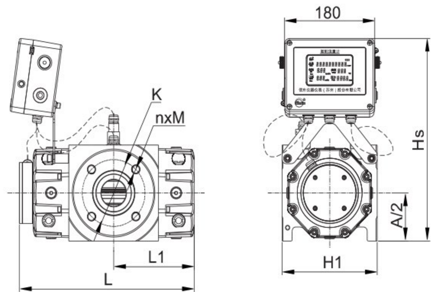
水平安装
