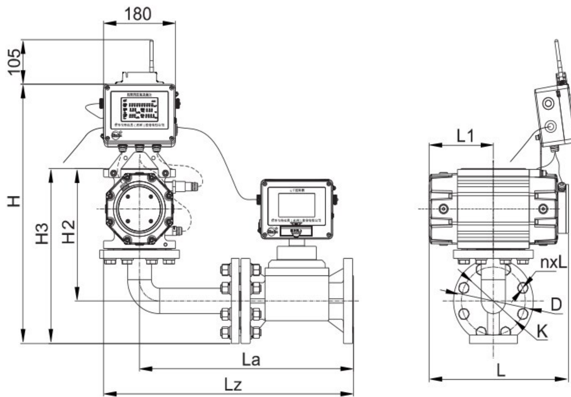
垂直安装
