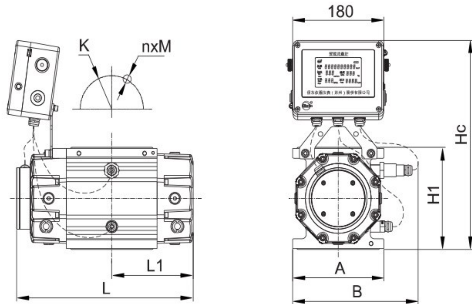
垂直安装
