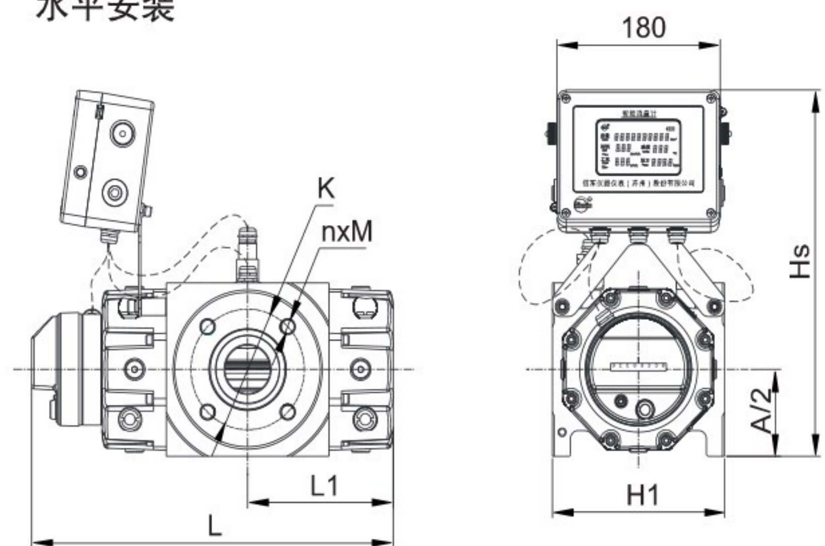
水平安装
