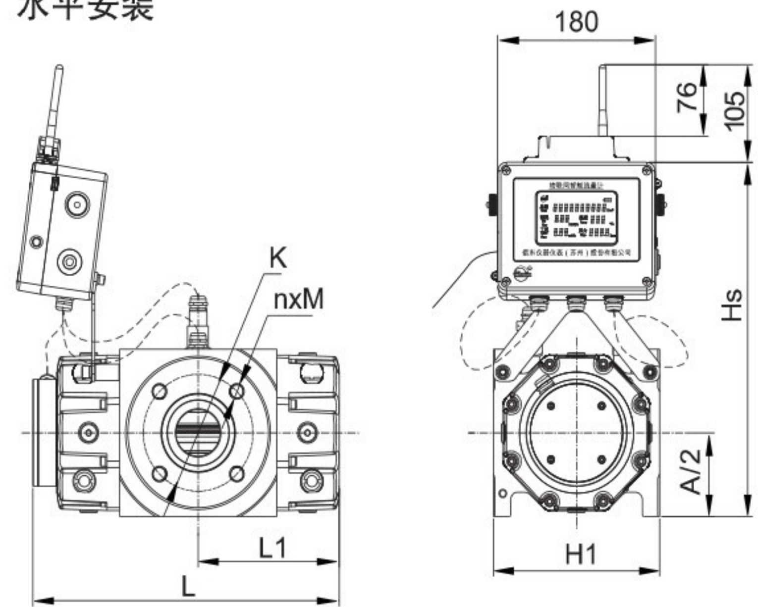
水平安装
