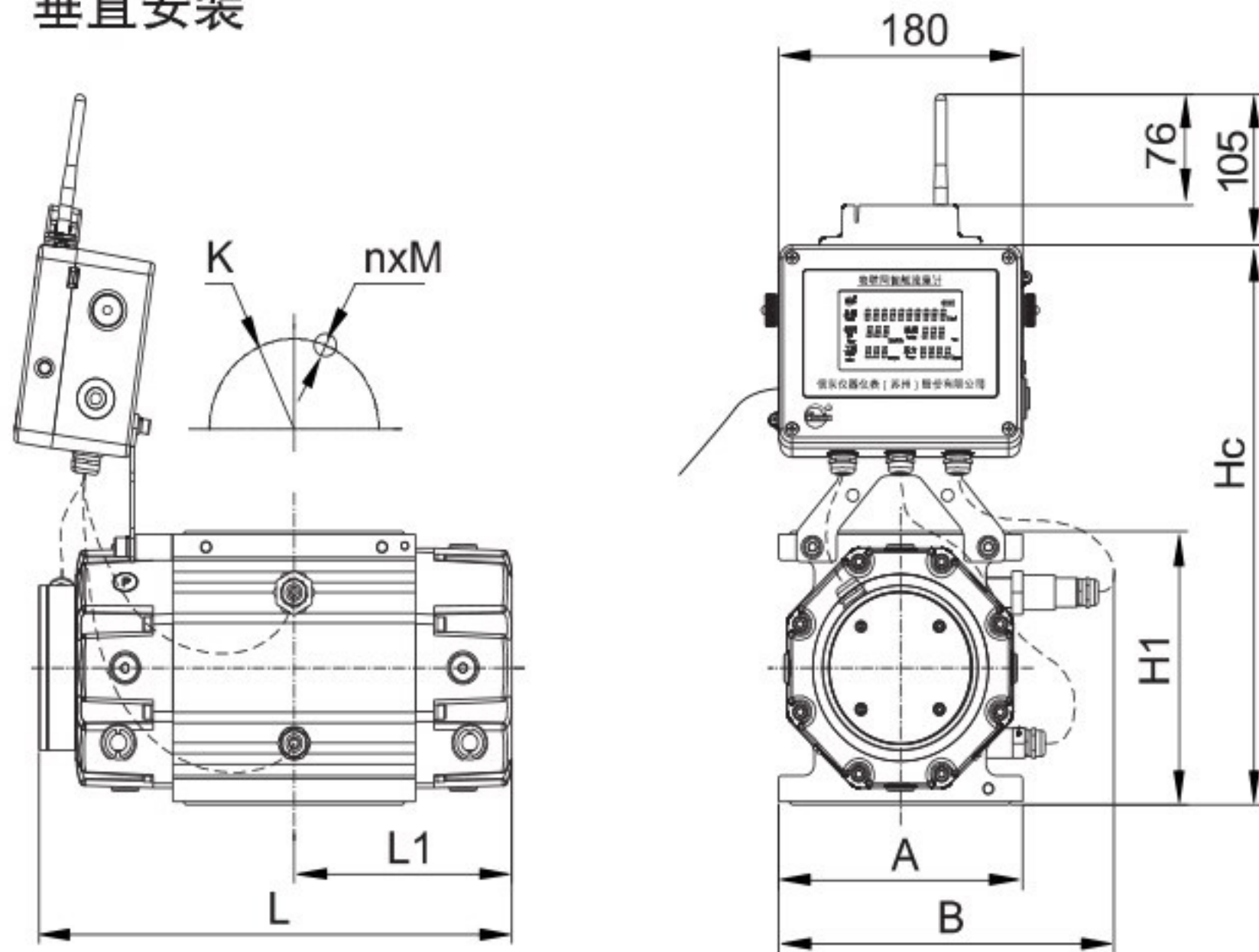
垂直安装
