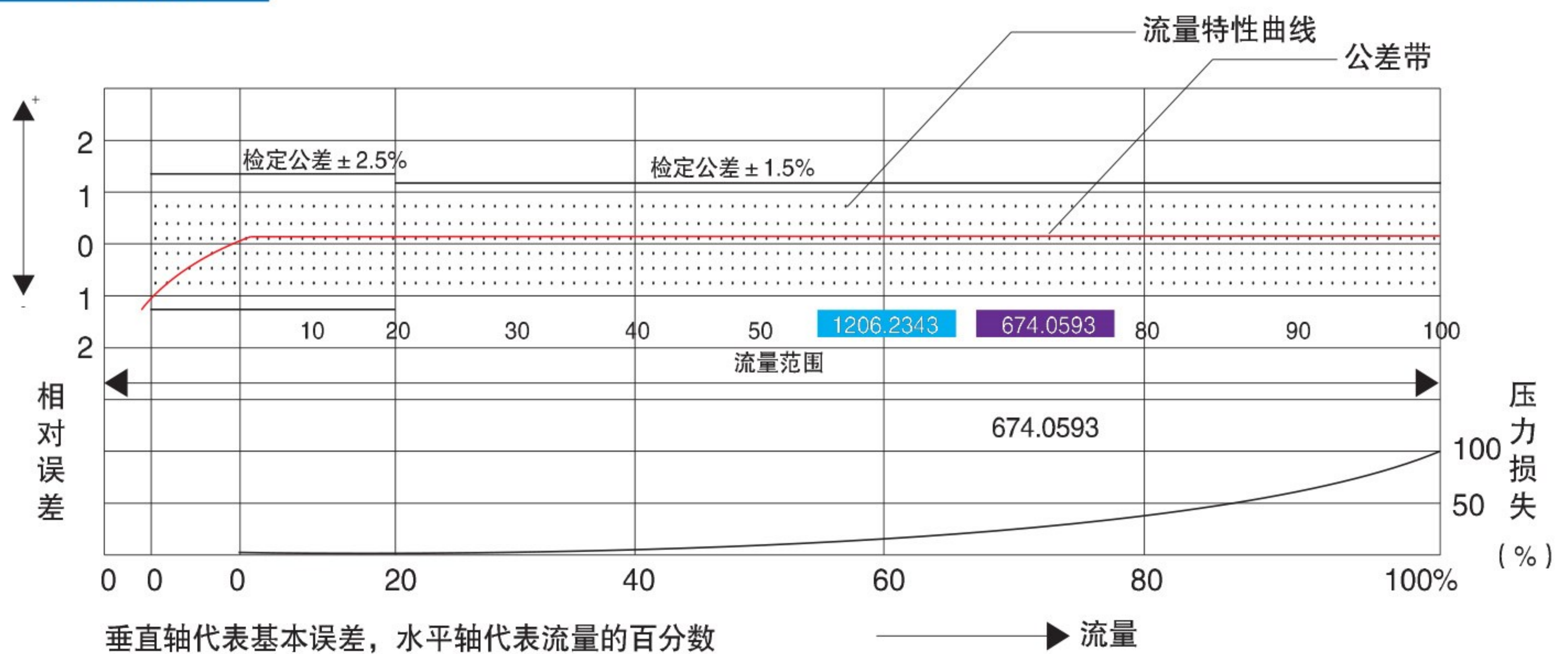
STLY典型误差曲线
