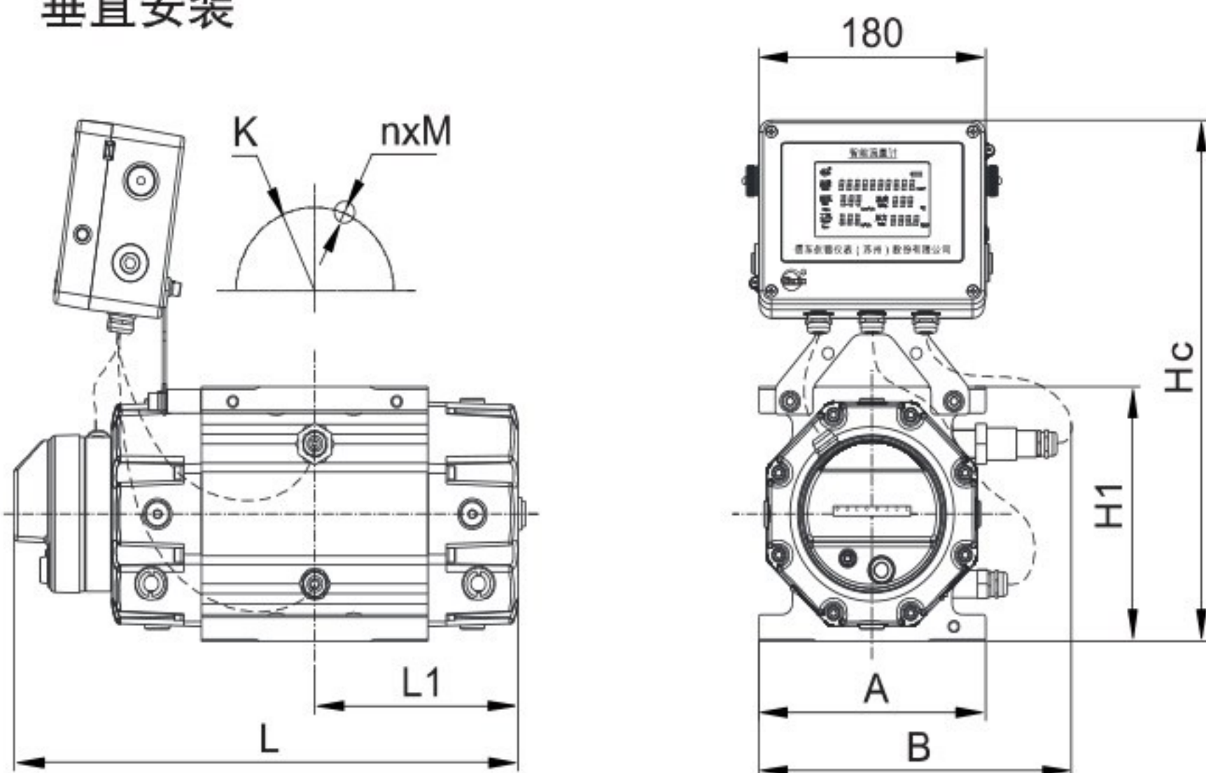
垂直安装
